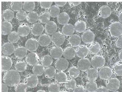
横断面(拡大)
